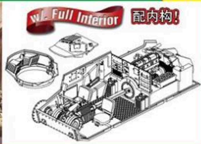
1:35 German Panzer Kpfw. 38(t) Ausf. B 德国Pz.Kpfw. 38(t) Ausf. B坦克 80141
