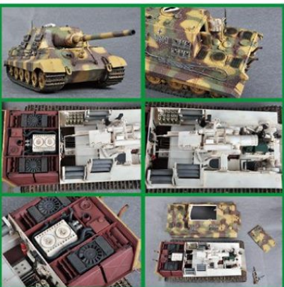
“猎虎”重型坦克歼击车
